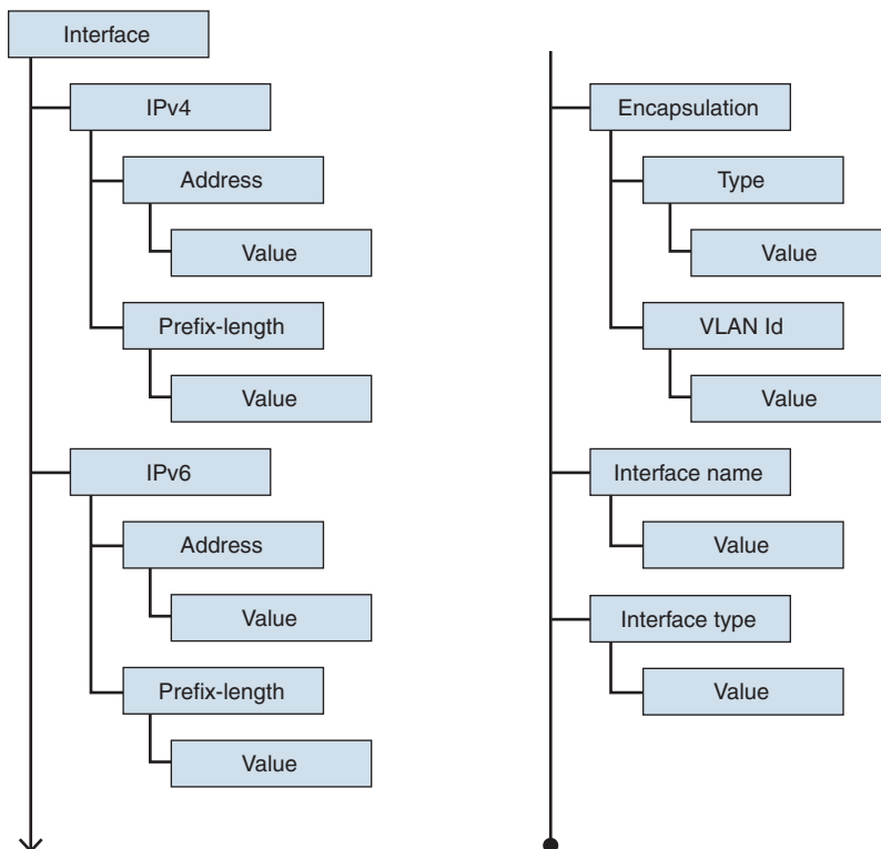
Figure 13-1 Generic Overview of a YANG Module
