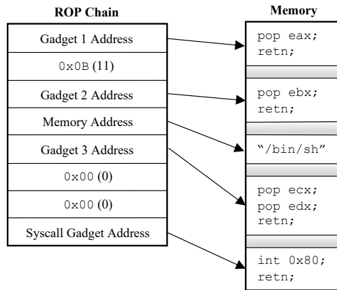
Fig. 1. Simple ROP Exploit Chain
