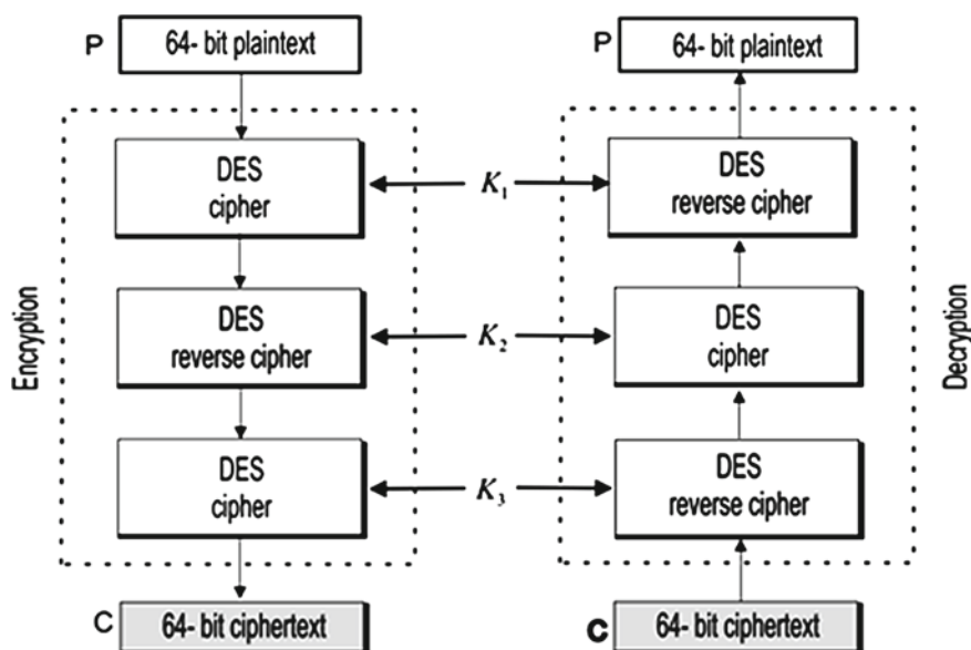
Fig. 3 DES algorithm
