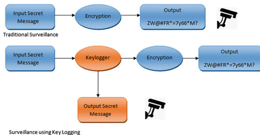
Fig. 14 Keylogger
