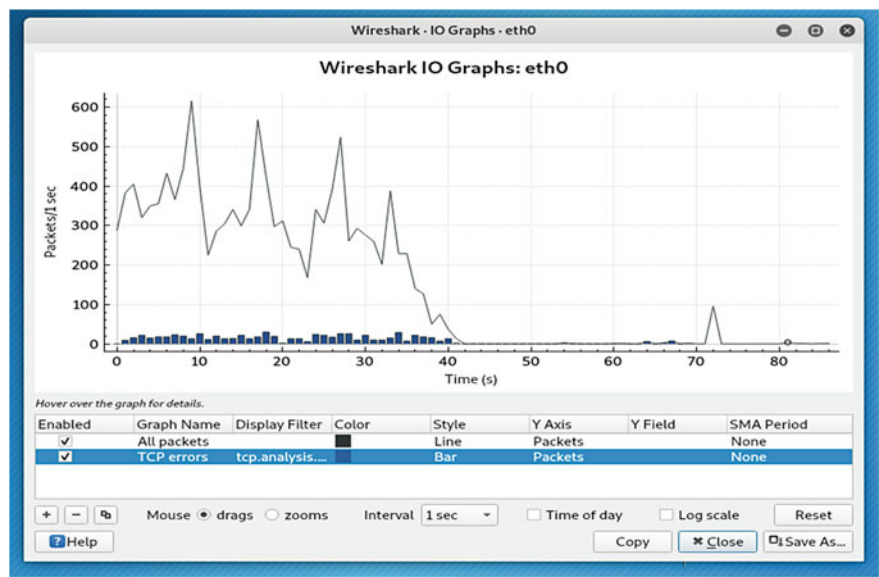
Fig. 2 DoS Attack
