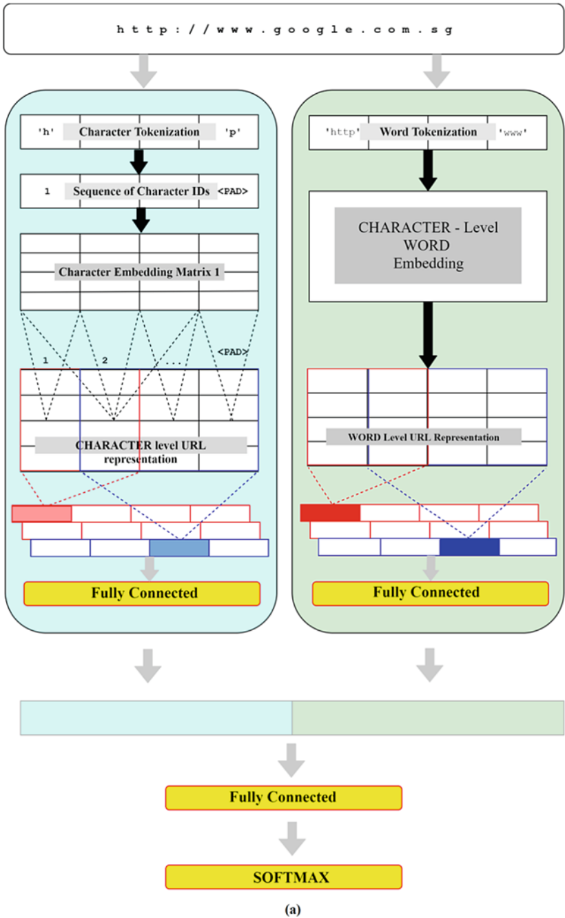
Fig. 8 URLNet
