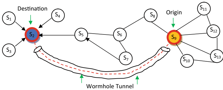
Fig. 3 Wormhole
