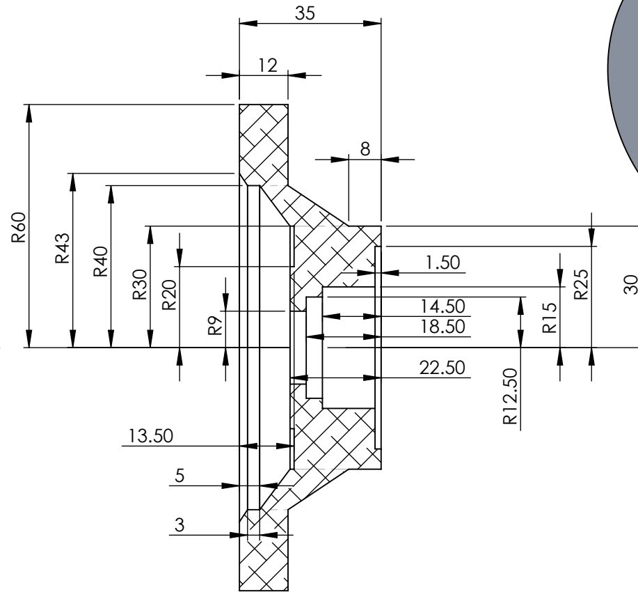
SECCIÓN A-A
