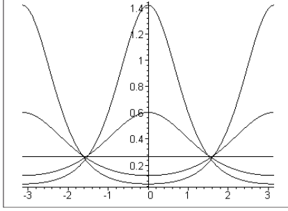
Figura 4: Q(8, \sigma) , \sigma = -0,1, -0,05, 0, 0,05 y 0,1
