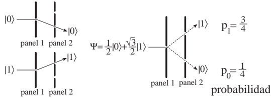
Figura 1: Medida del spin de \Psi = \frac{1}{2}|0\rangle + \frac{\sqrt{3}}{2}|1\rangle
