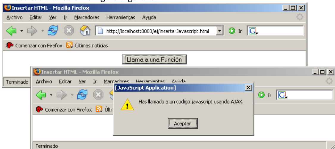
Ilustración 39 Código JavaScript devuelto por AJAX y evaluado.
