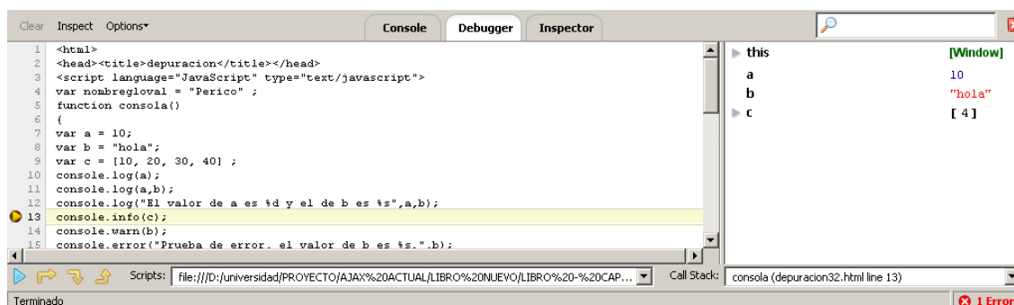
Ilustración 30 Pestaña de debugger de FireBug con un punto de ruptura.
