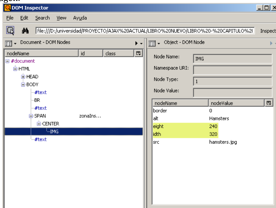
Ilustración 18 Ejemplo de uso de la utilidad DOM inspector.
