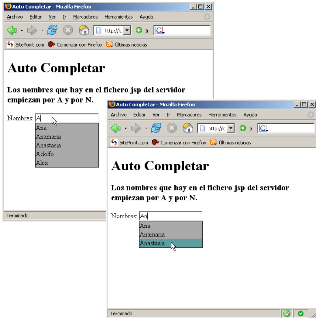
Ilustración 62 Ejemplo de auto completado empleando AJAX.
