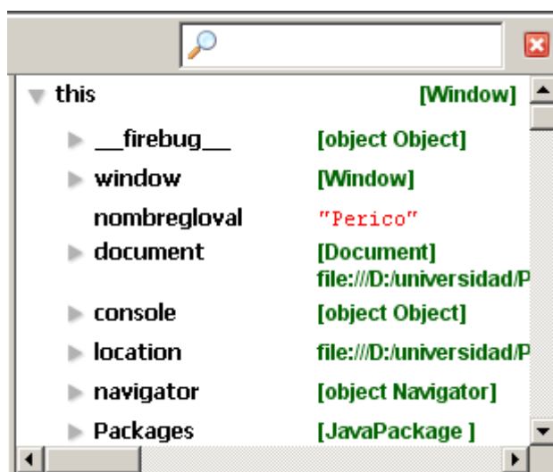
Ilustración 31 Mostrando el árbol de objetos JavaScript del DOM con FireBug.
