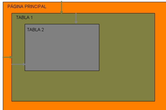
Ilustración 59 Tablas anidadas.
