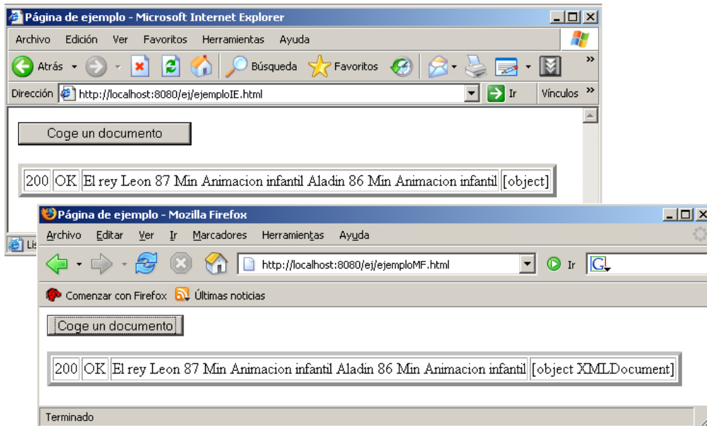
Ilustración 7 Propiedades del objeto mostradas en Internet Explorer y Mozilla Firefox.
