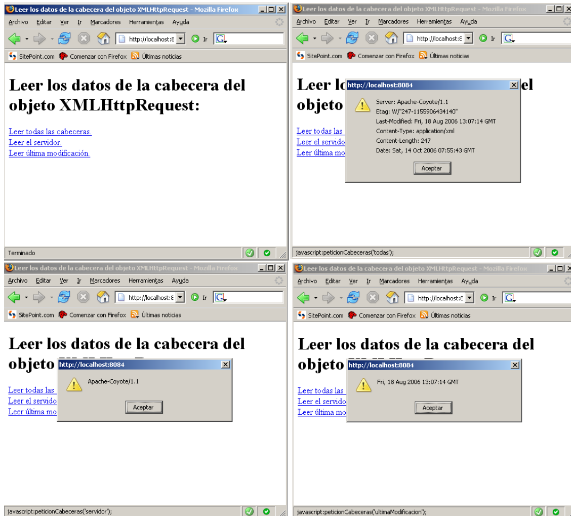
Ilustración 50 Ejemplo de leer las cabeceras del objeto XMLHttpRequest.
