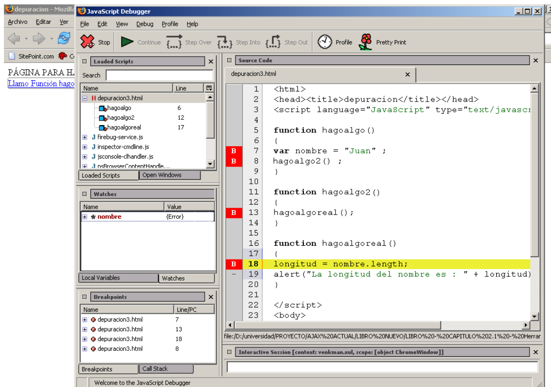
Ilustración 23 Estado tras el paso 7 de la explicación.
