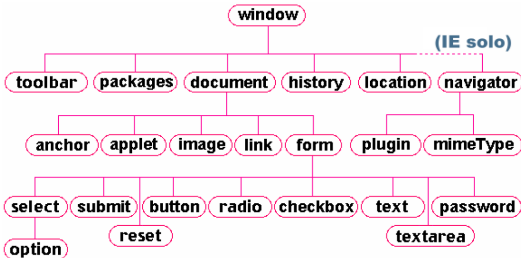
Ilustración 42 Jerarquía de objetos del navegador.
