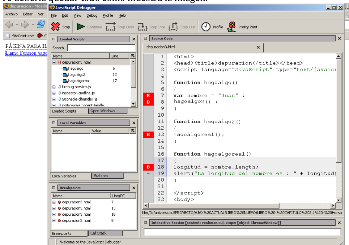
Ilustración 20 Venkman con el fichero depuracion3.html cargado, después de poner algunos breakpoints.
