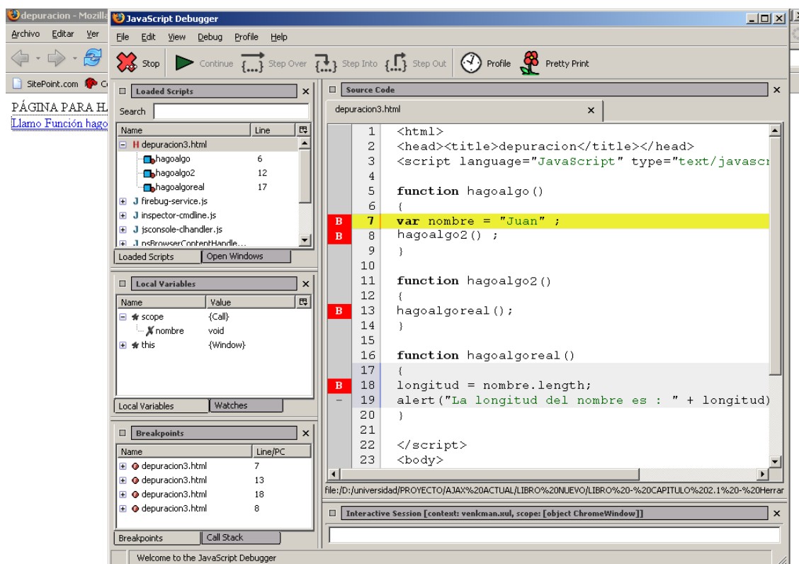
Ilustración 21 Venkman con el fichero depuracion3.html cargado, detenido por un punto de ruptura.
