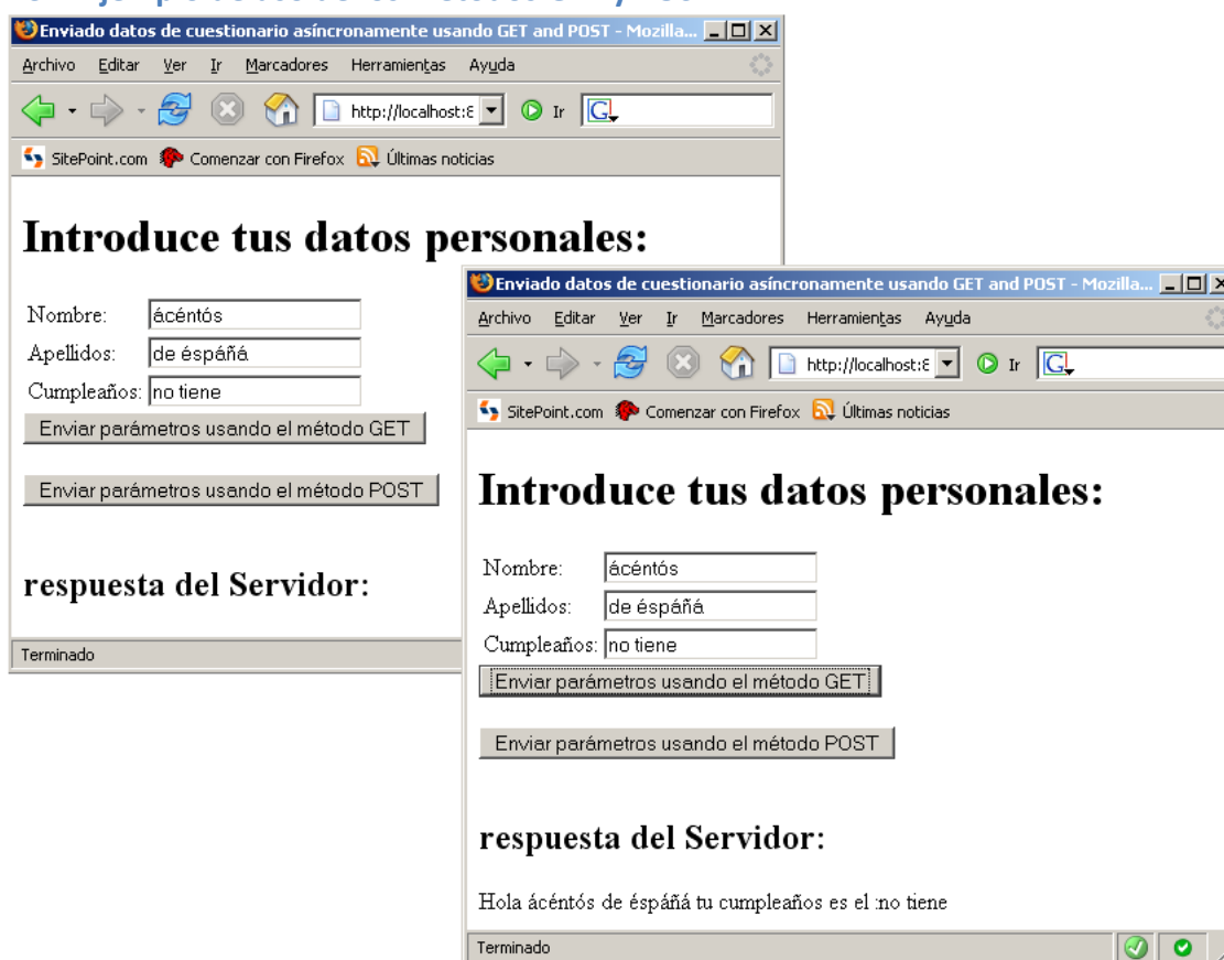
Ilustración 49 Ejemplo de los métodos GET y POST.
