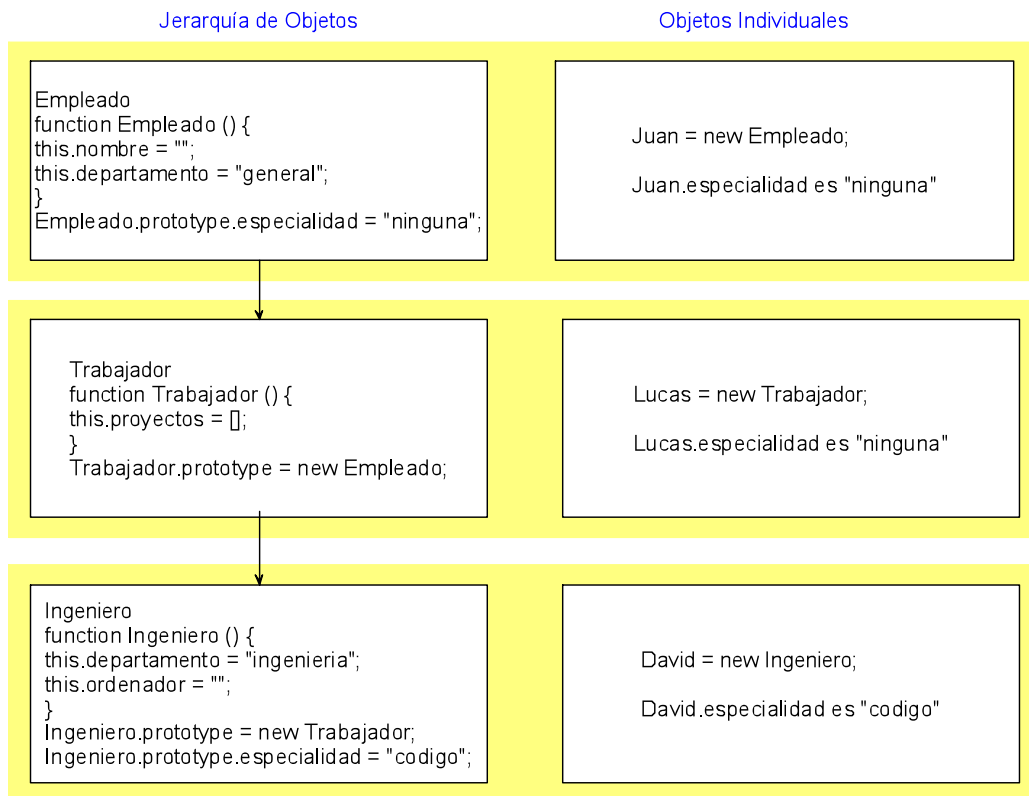
Ilustración 12 Ejemplo de uso de prototipos, traducido de "Core JavaScript Guide".
