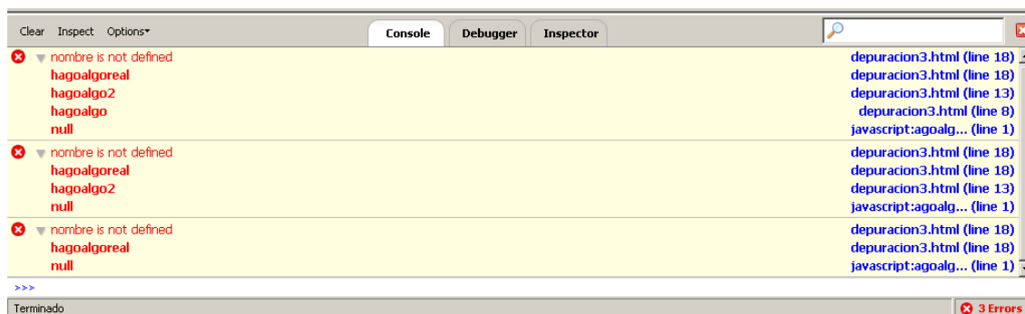
Ilustración 28 Pila de llamadas de los errores mostrados en la consola de FireBug.
