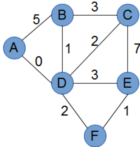
ILUSTRACIÓN 8 - Grafo del ejercicio 2.
