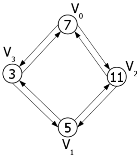
Figura 12.14: Grafo fuertemente conexo.
