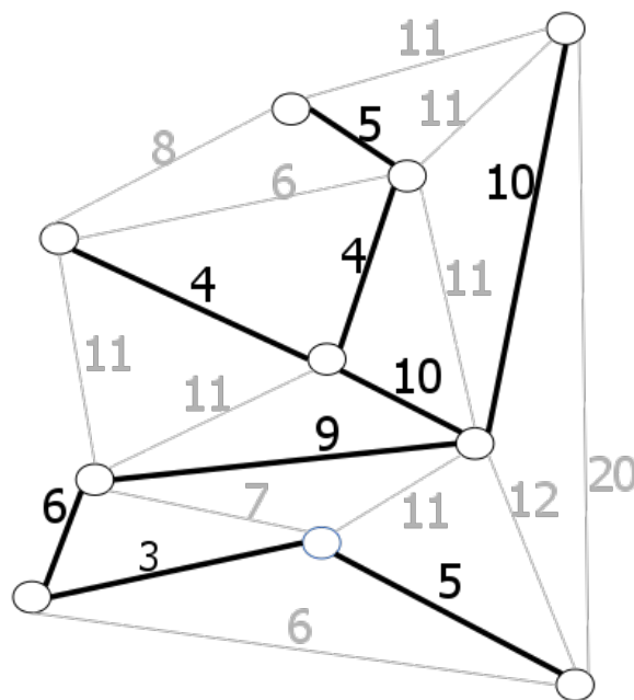
Figura 12.23: Árbol de expansión mínima
