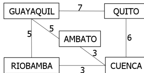
Figura 12.8: Explicación del factor de peso, distancia entre ciudades.
