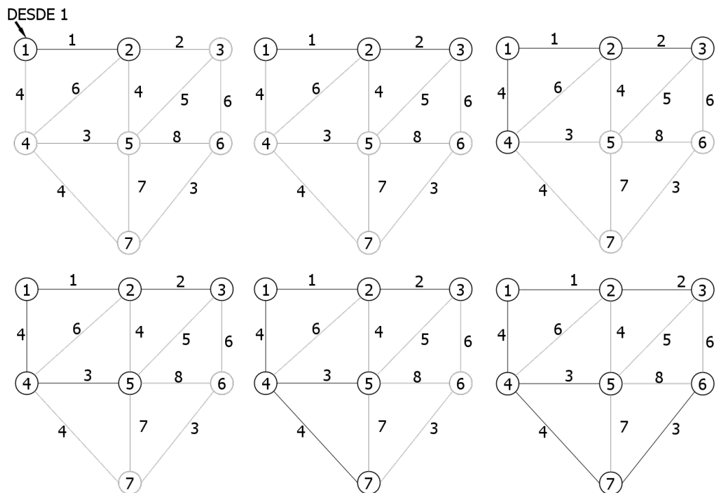
Figura 12.25: Pasos del algoritmo de Prim.
