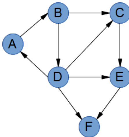
ILUSTRACIÓN 9 - Grafo del ejercicio 3.
