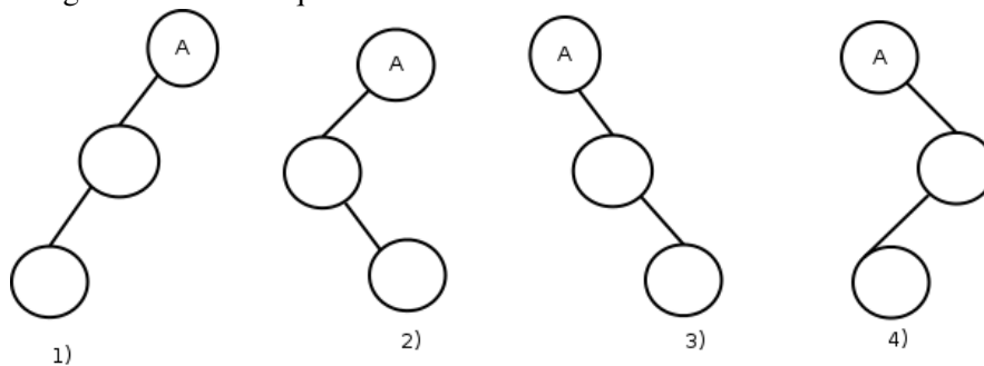
Figura 10.2: Casos que se deben tener en cuenta al reestructurar un nodo
