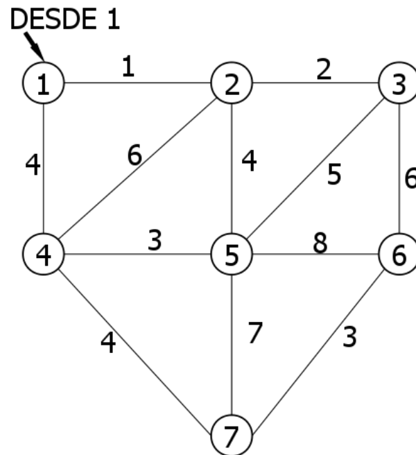
Figura 12.24: Grafo conexo, no dirigido. Ejemplo empleado para extraer el árbol de expansión mínima.
