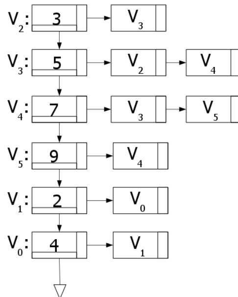
Figura 12.18: Representación de la lista de adyacencia consecuente al grafo de la figura 12.16
