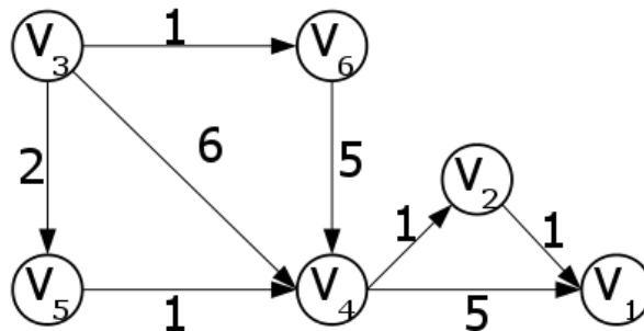
Figura 12.22: Grafo dirigido con factor de peso, ejemplo empleado en el desarrollo del Algoritmo de Dijkstra
