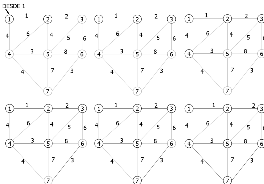
Figura 12.26: Pasos del algoritmo de Kruskal
