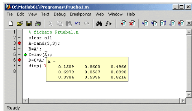
Figura 17. Ejecución interactiva con el Editor/Debugger.
