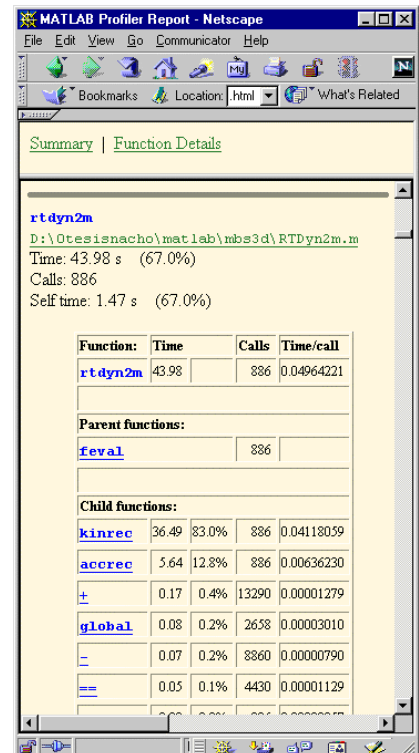
Figura 30. Informe sobre una función.
