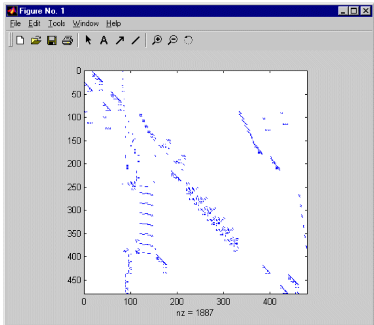
Figura 24. Ejemplo de matriz dispersa (west0479).
