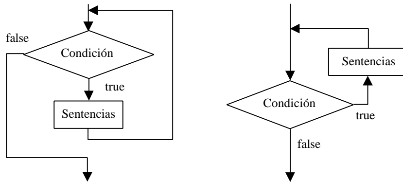
Figura 26. Bucles con control al principio y al final.
