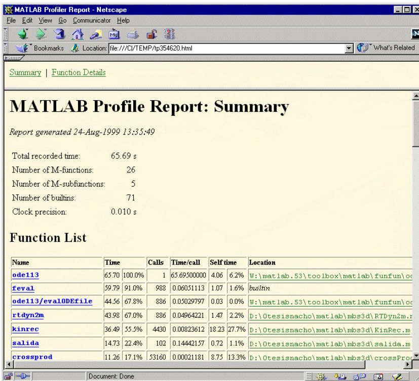
Figura 29. Página principal del informe del profiler.
