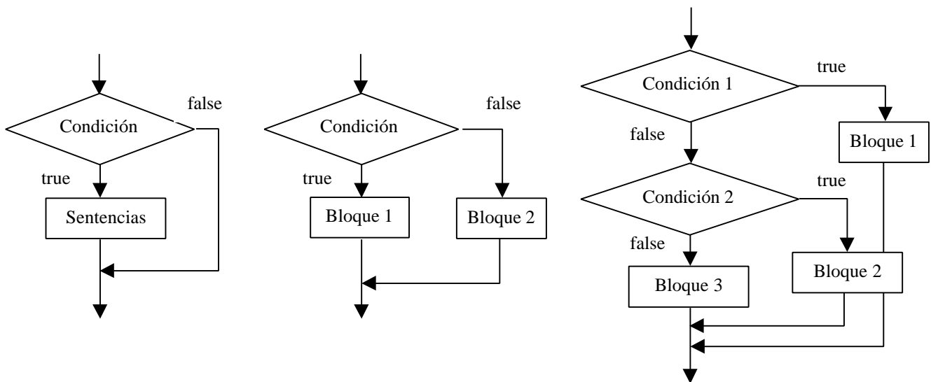
Figura 25. Ejemplos gráficos de bifurcaciones.
