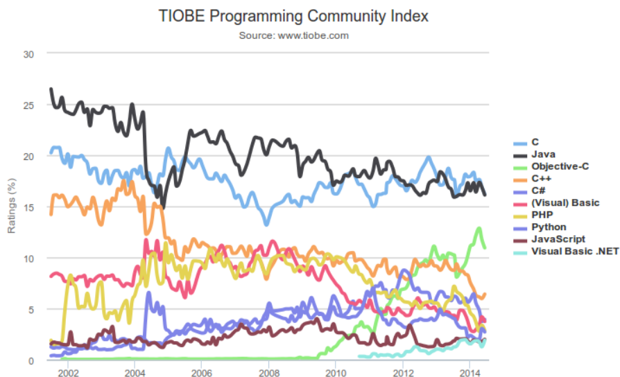
Figure 4.1: TIOBE Index 2002–2014
